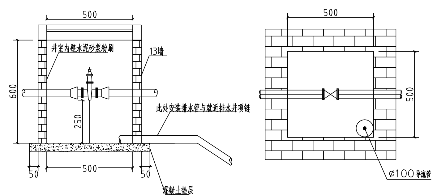
Z-50及以下阀门井室图例
