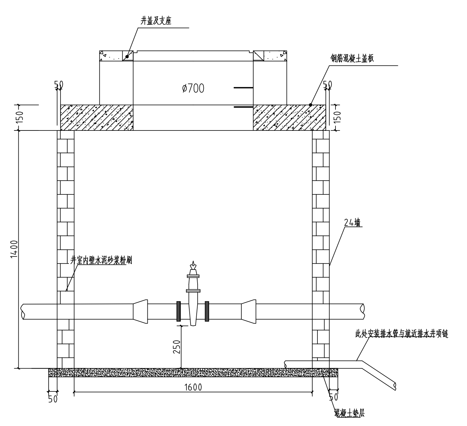
Z-300阀门井室（直筒井）图例
