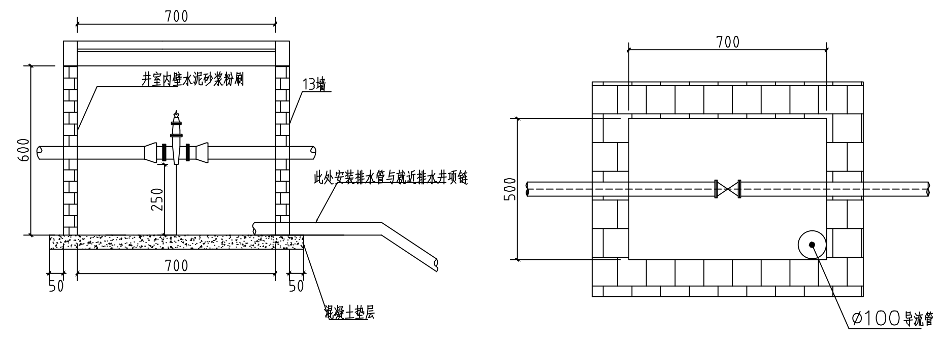
Z-65阀门井室图例
