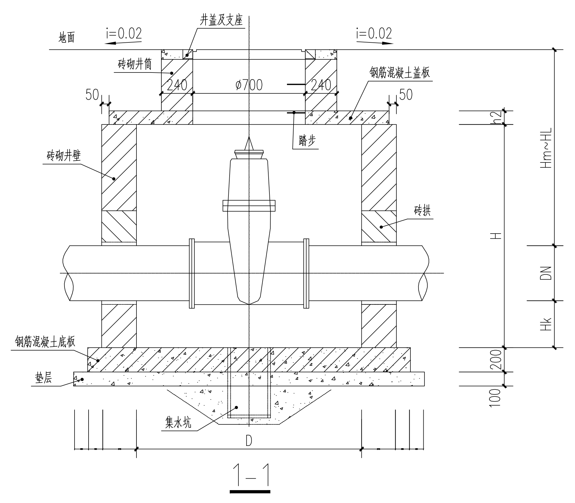
Z-80、100阀门井室图例
