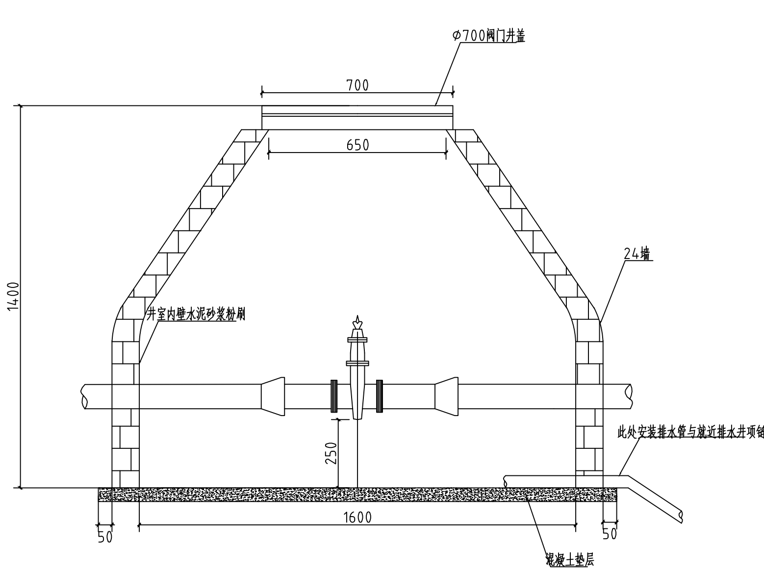
Z-250阀门井室图例
