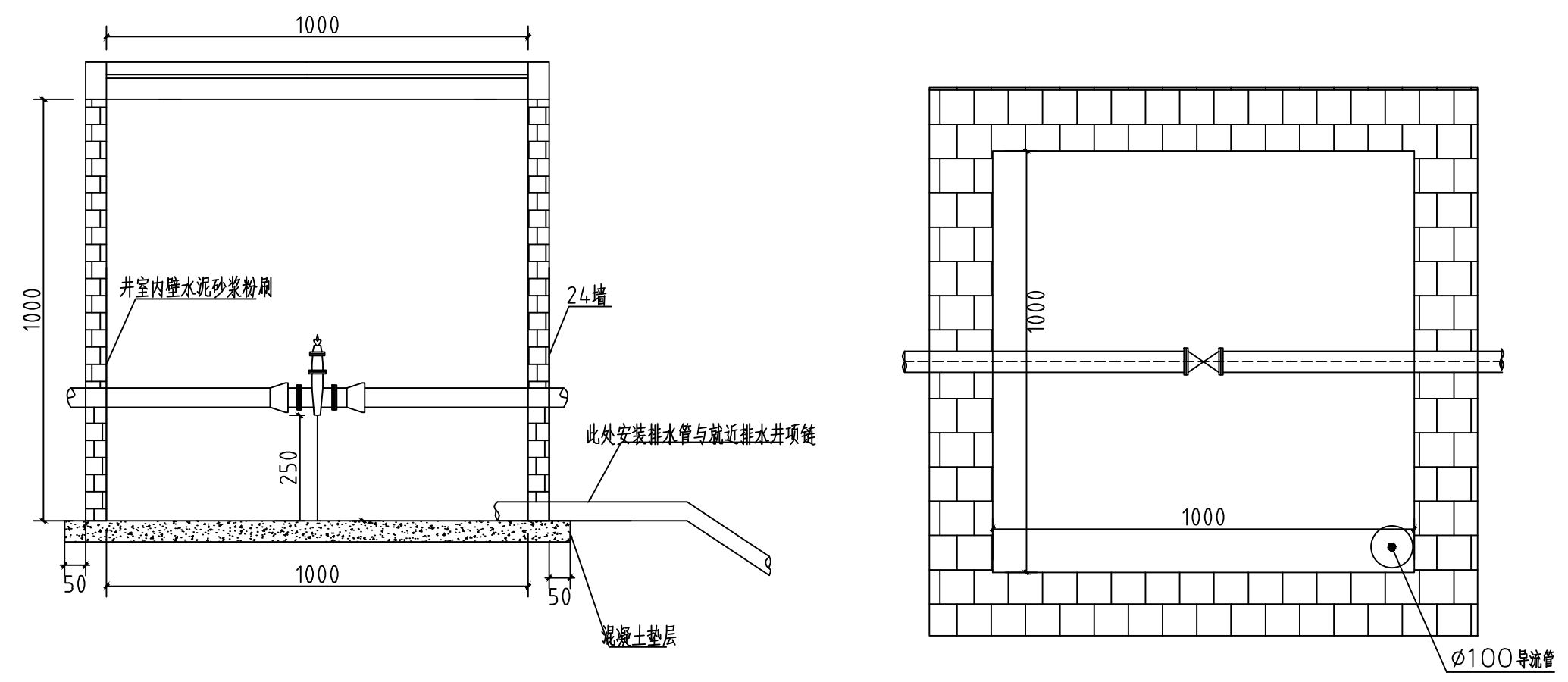
Z-80、100阀门井室图例
