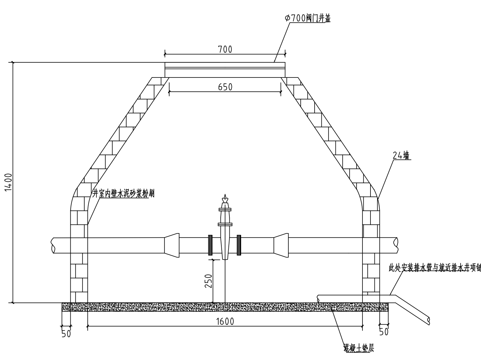
Z-300阀门井室图例
