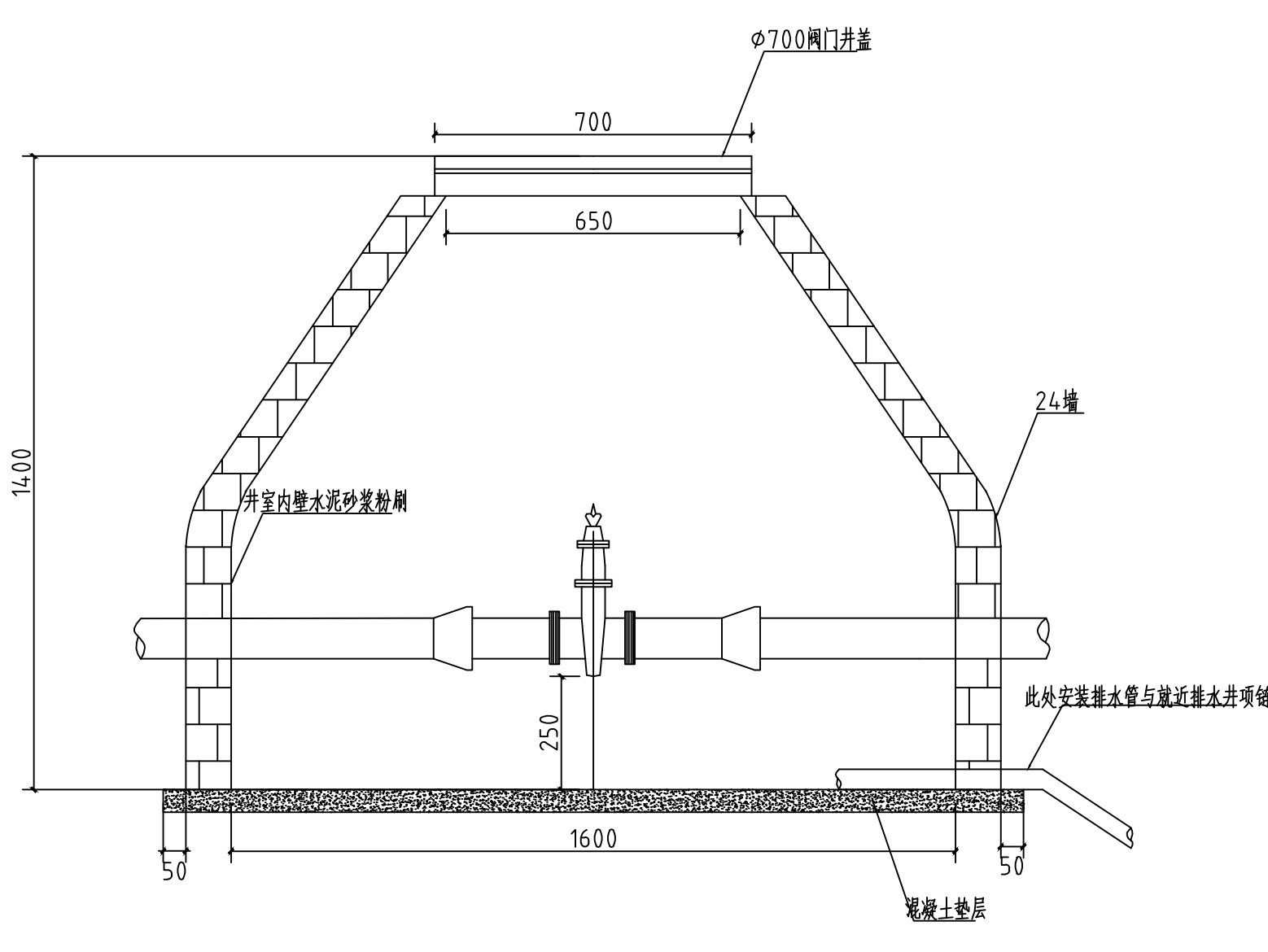
Z-200阀门井室图例
