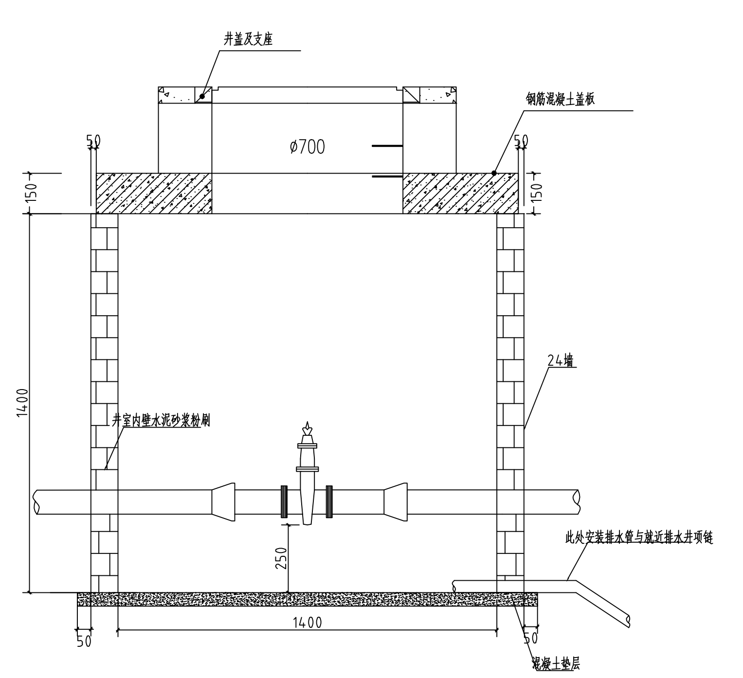
Z-250阀门井室（直筒井）图例
