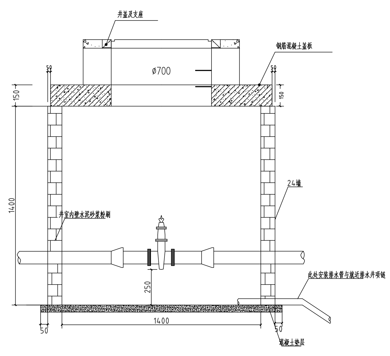
Z-200阀门井室（直筒井）图例
