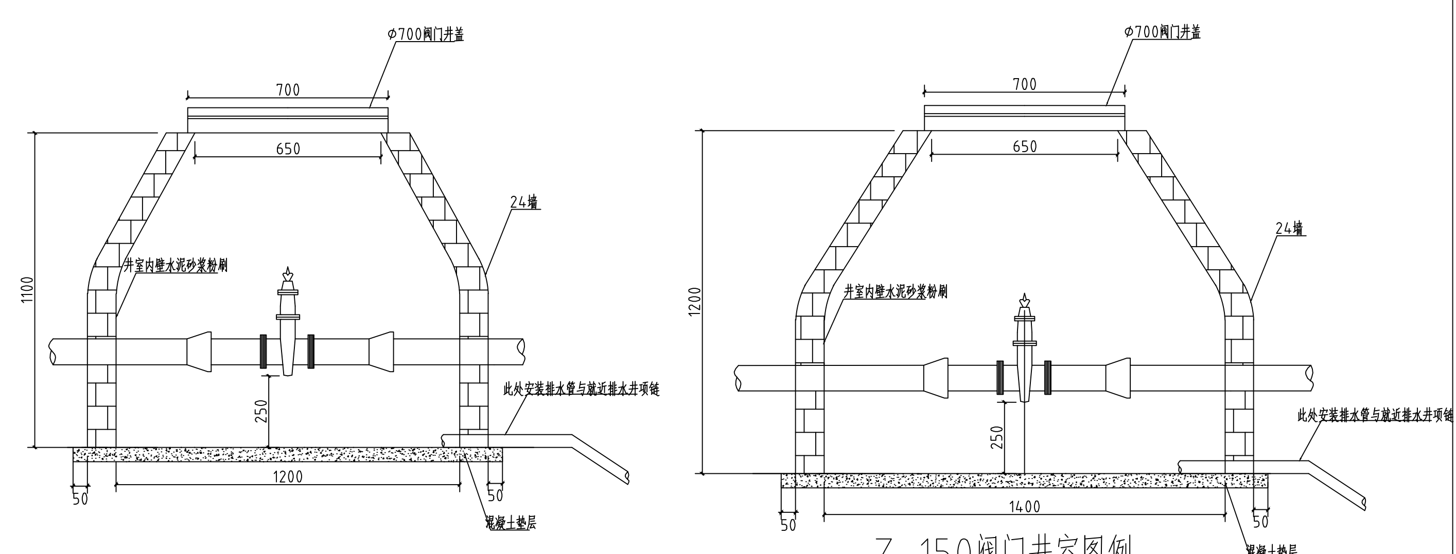
Z-150阀门井室图例
