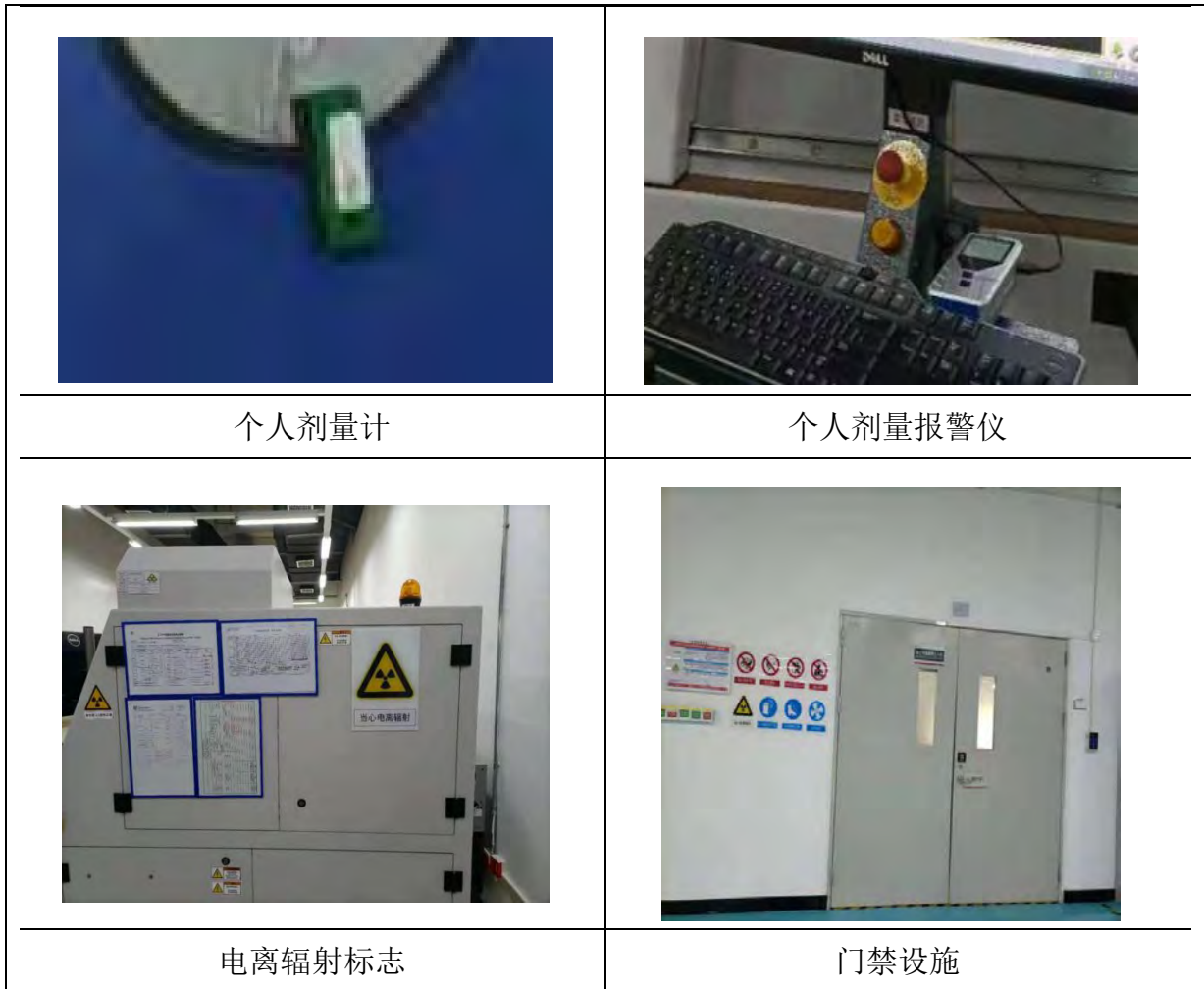
图 4-1 辐射安全与防护设施实物图
