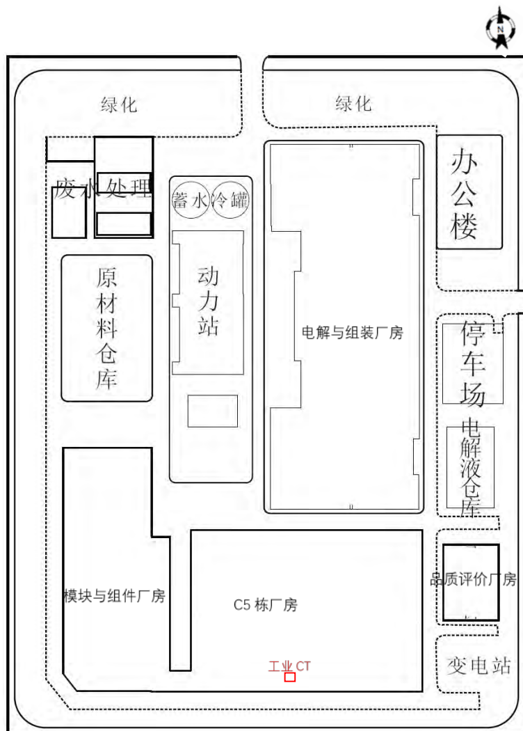
图 2-1 亿纬集能厂区平面布置图
