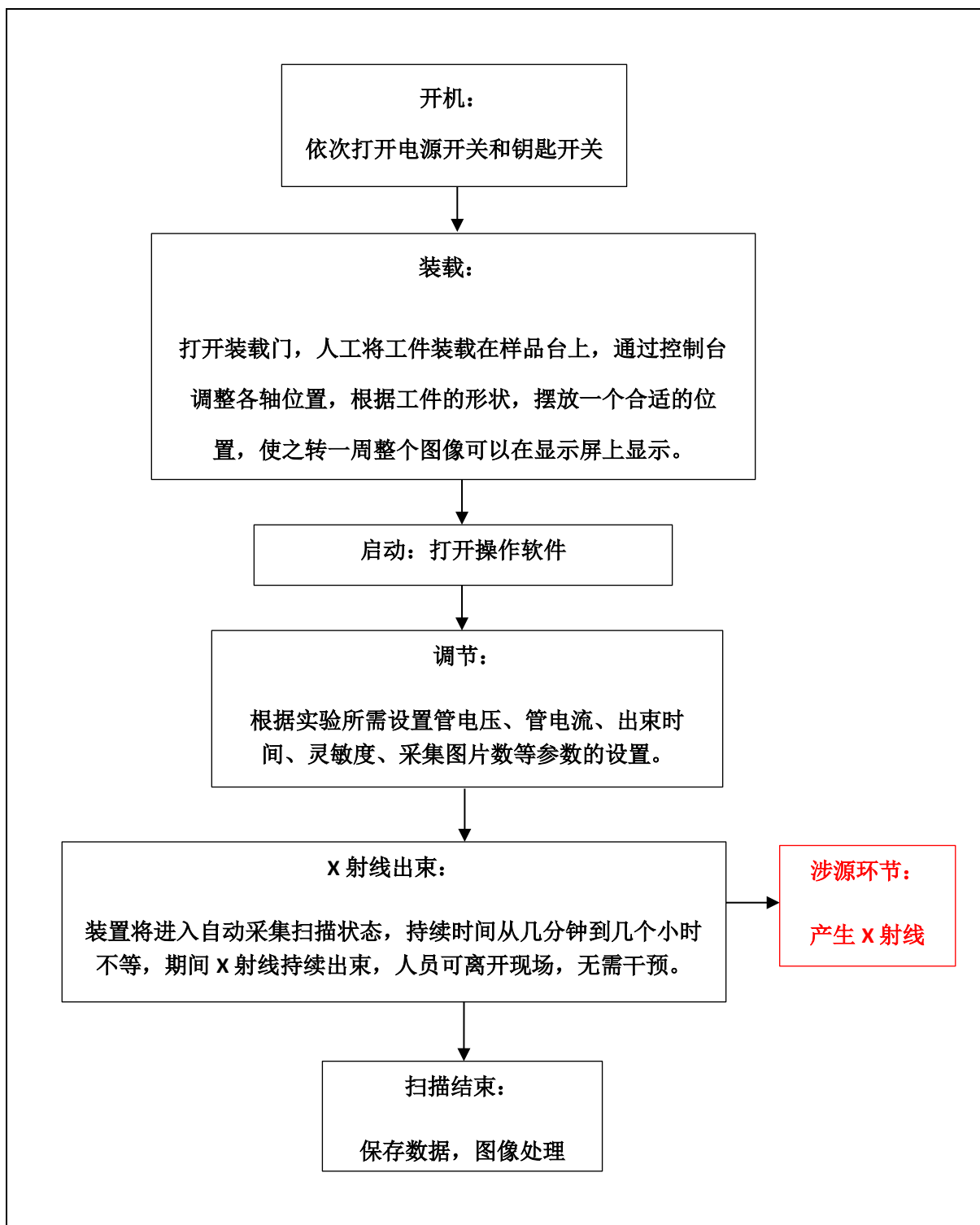
图 3-4 装置操作流程图
