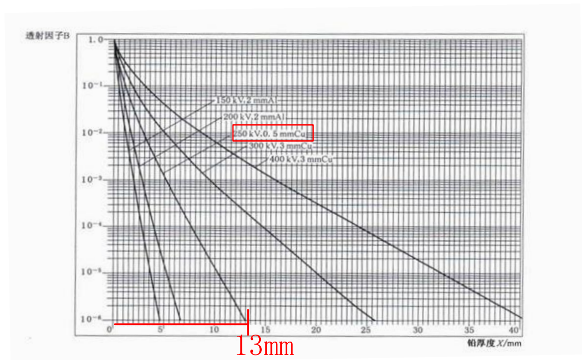
图 11-3 X 射线穿过铅的透射因子
