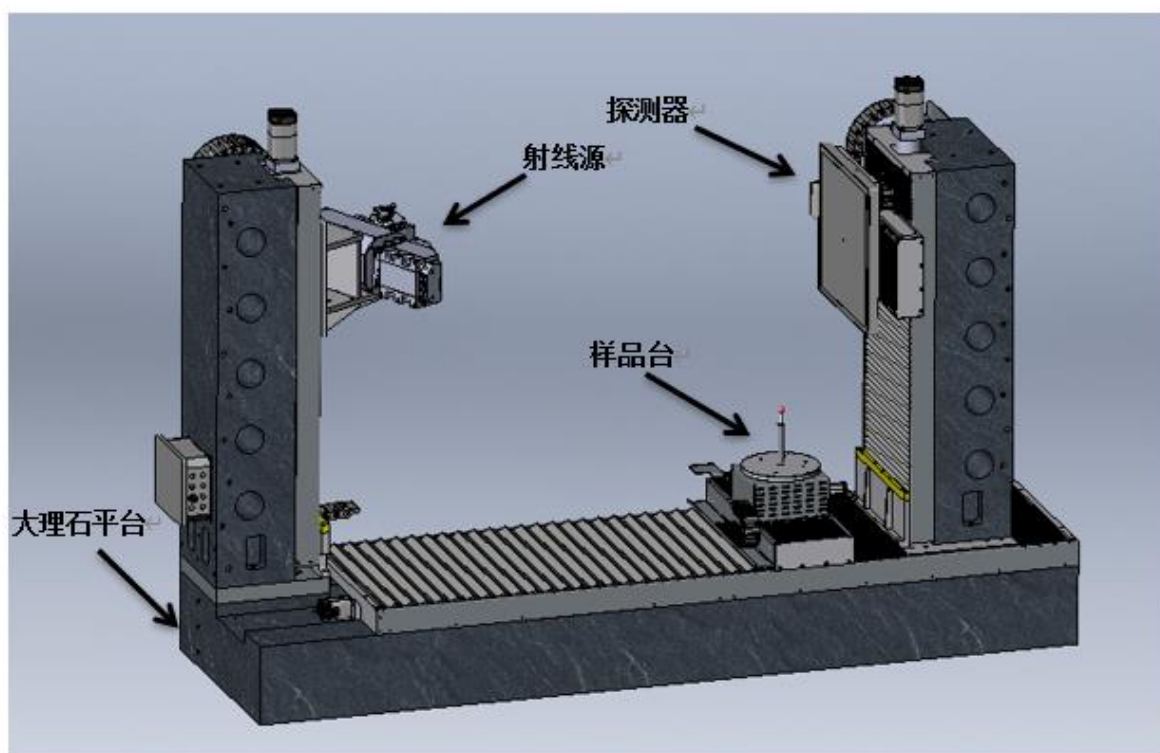
图 9-3 设备内部结构图
