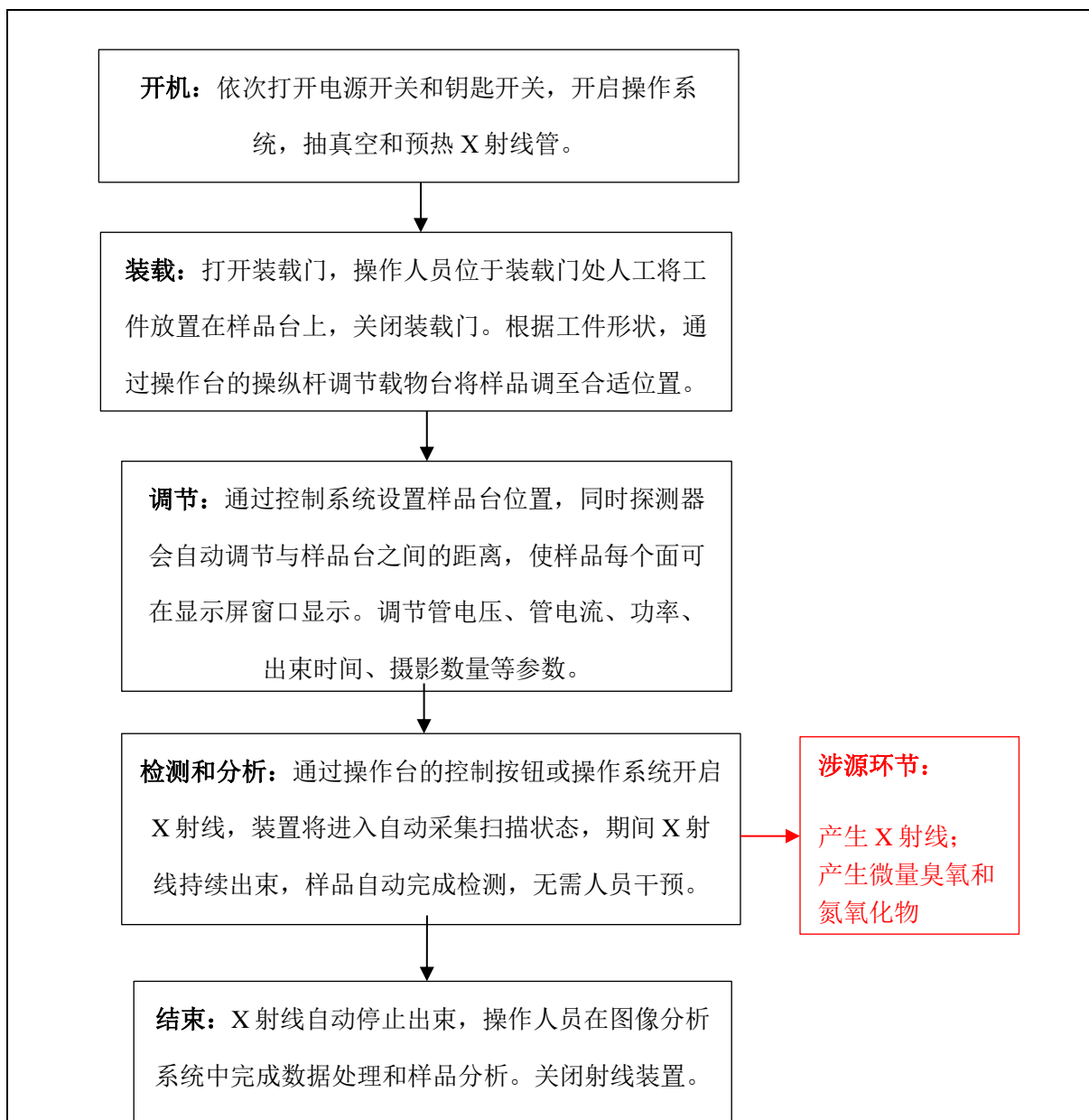
图 9-4 工艺流程和产污环节图
