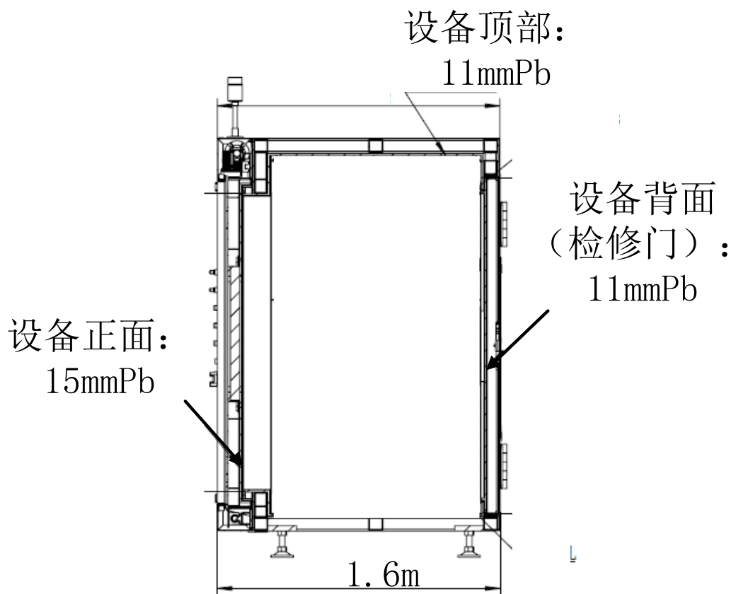
图 10-2 射线装置右视图
