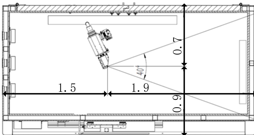
俯视图
