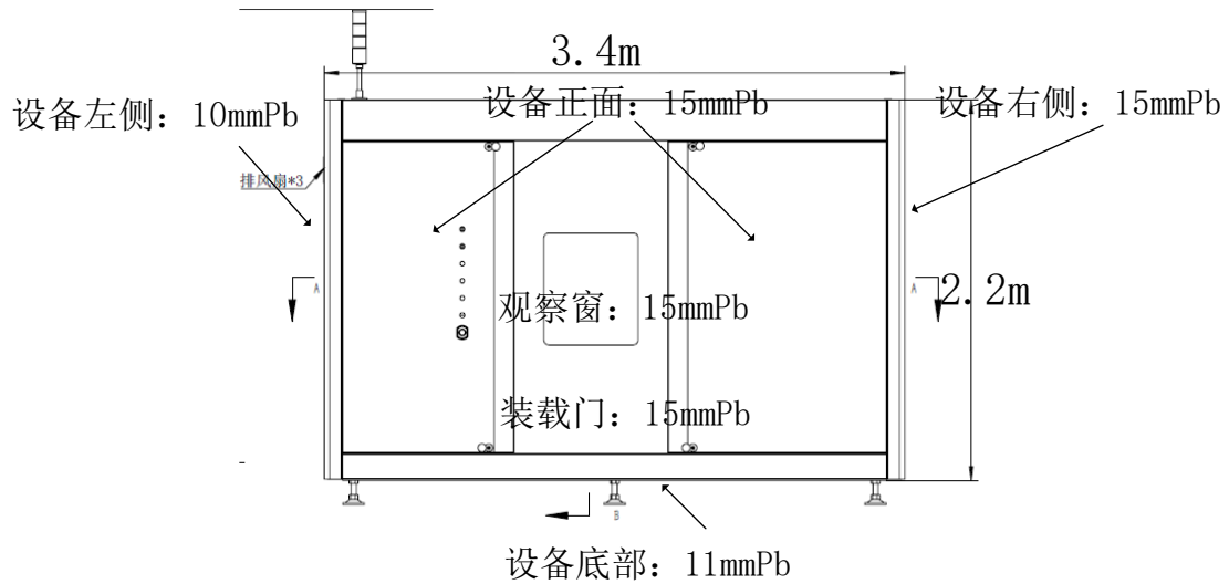
图 10-1 射线装置正视图
