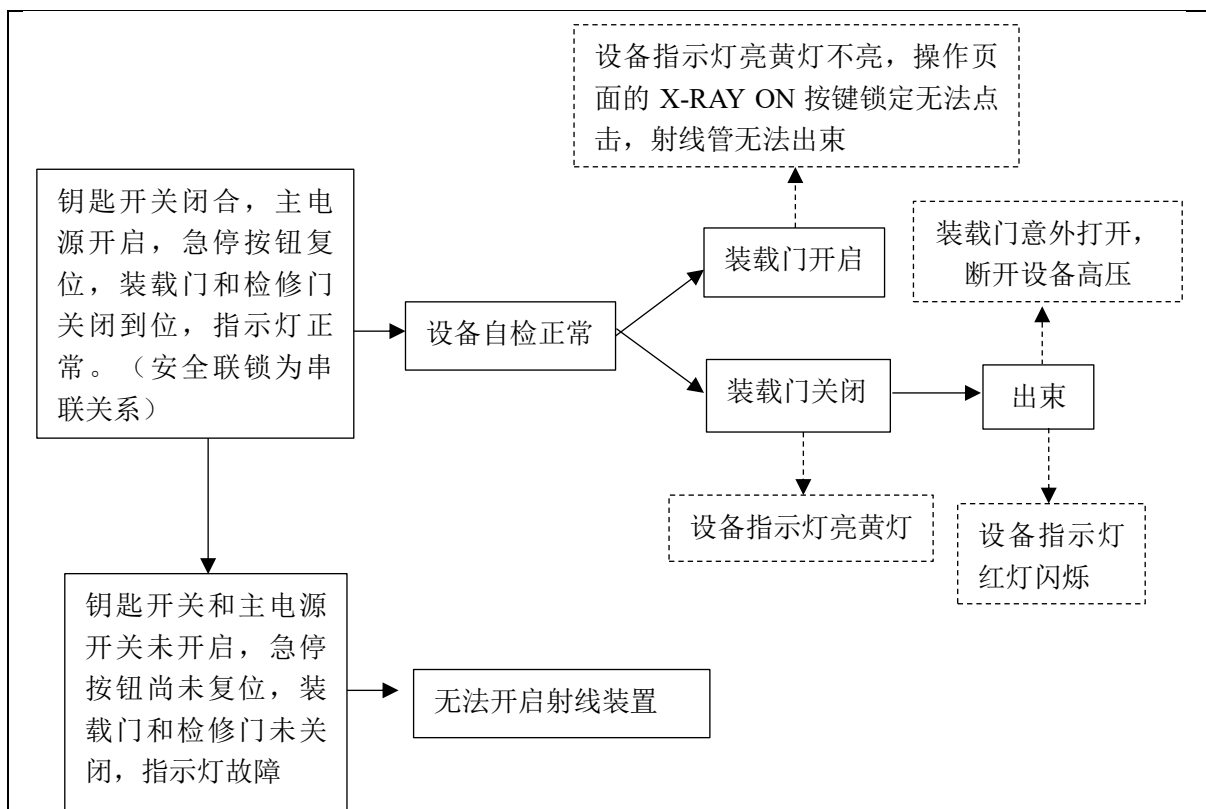
图 10-6 门机联锁逻辑图
