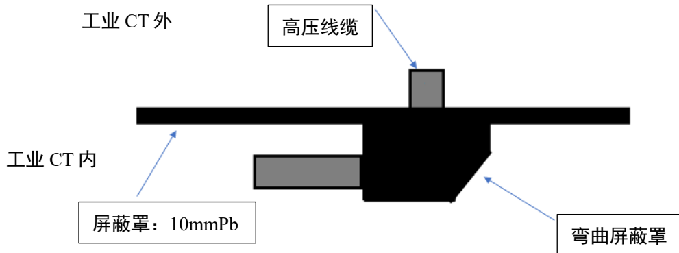
图 10-3 管线穿屏蔽体示意图
