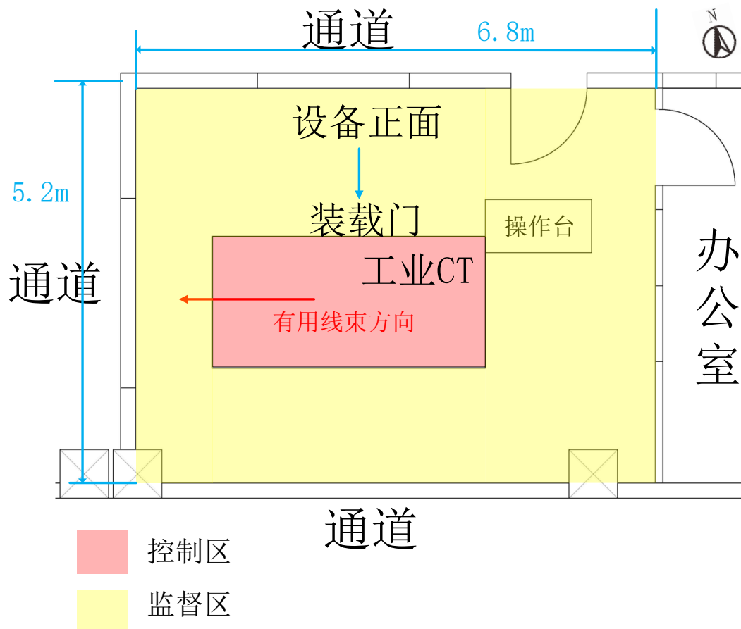
图 10-7 辐射工作场所布局和分区示意图
