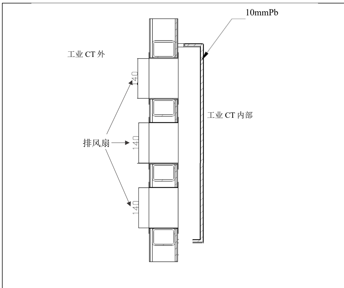
图 10-4 排风口屏蔽示意图
