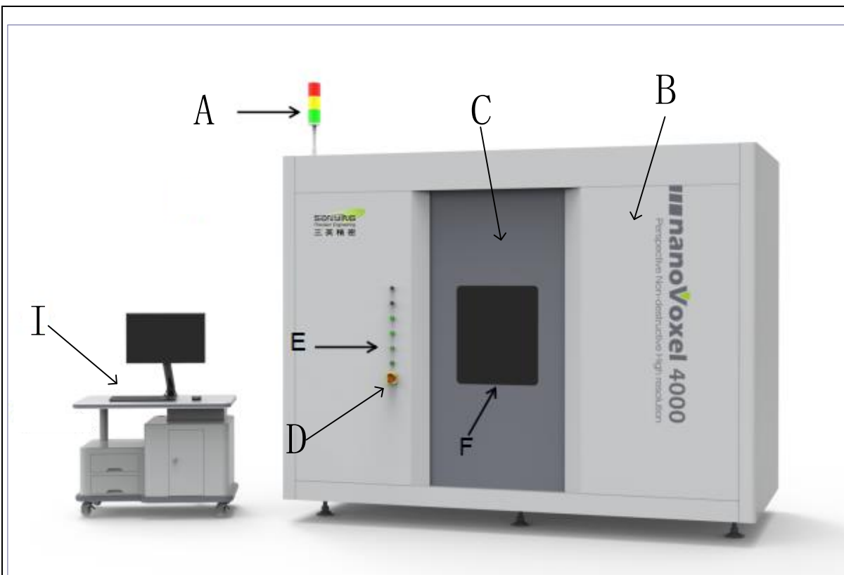
图 9-2 设备外观结构图
