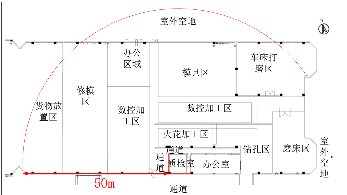
图 1-3 B 栋车间 1 楼平面图
