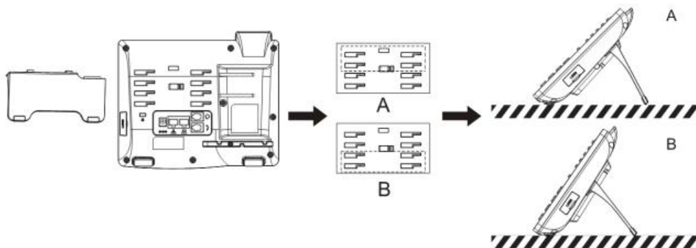
图 4 - GW26G 桌面式话机安装
