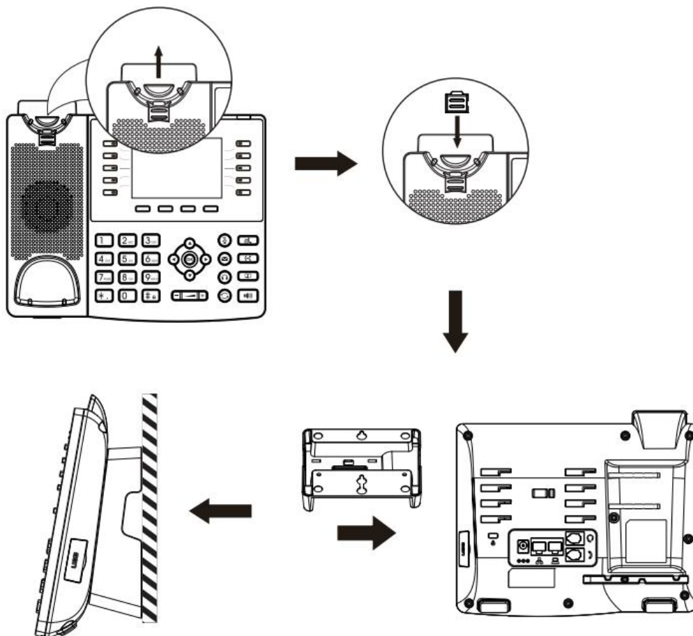
图 5 - GW26G 壁挂式安装
