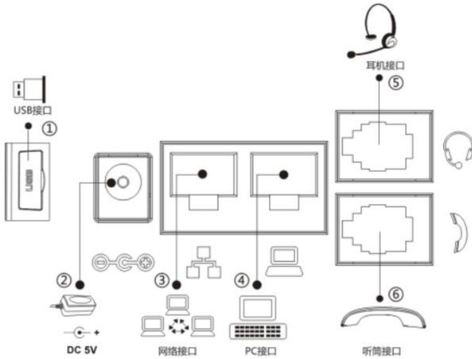
图 6 - GW26G 设备连接
