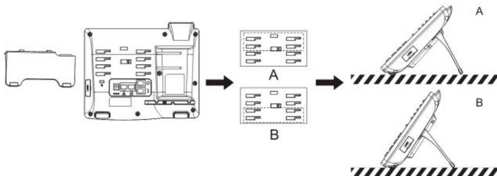
图 1 - GW23G 桌面式话机安装
