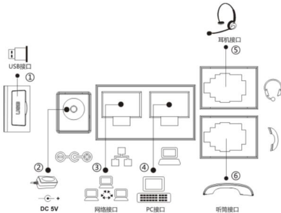
图 3 - GW23G 设备连接
