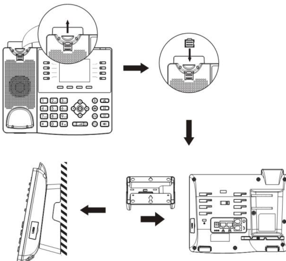
图 2 - GW23G 壁挂式安装
