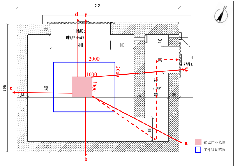
图 11-1 本项目探伤室平面布局与预测点位图（单位:mm）
