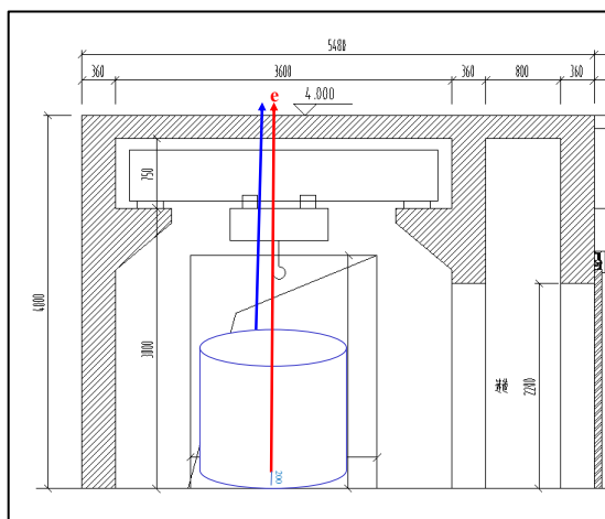
图 11-2 本项目探伤室剖面布局与预测点位图（单位:mm）
