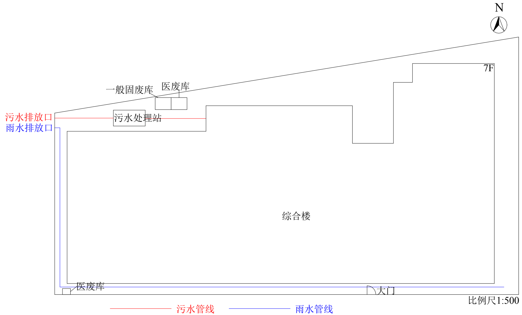
图 3-3 平面布置图
